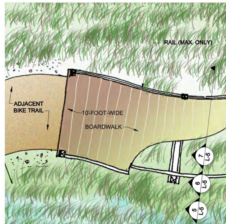
2 BOARDWALK (MOD./MAX.) L-5 SCALE: NTS
