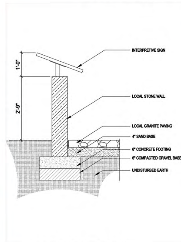
6 VIEW POINT (MAX.) L-3 SCALE: NTS
