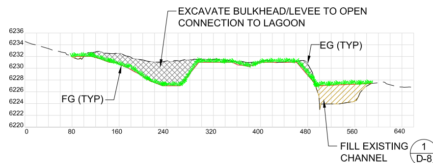
SECTION D-D
